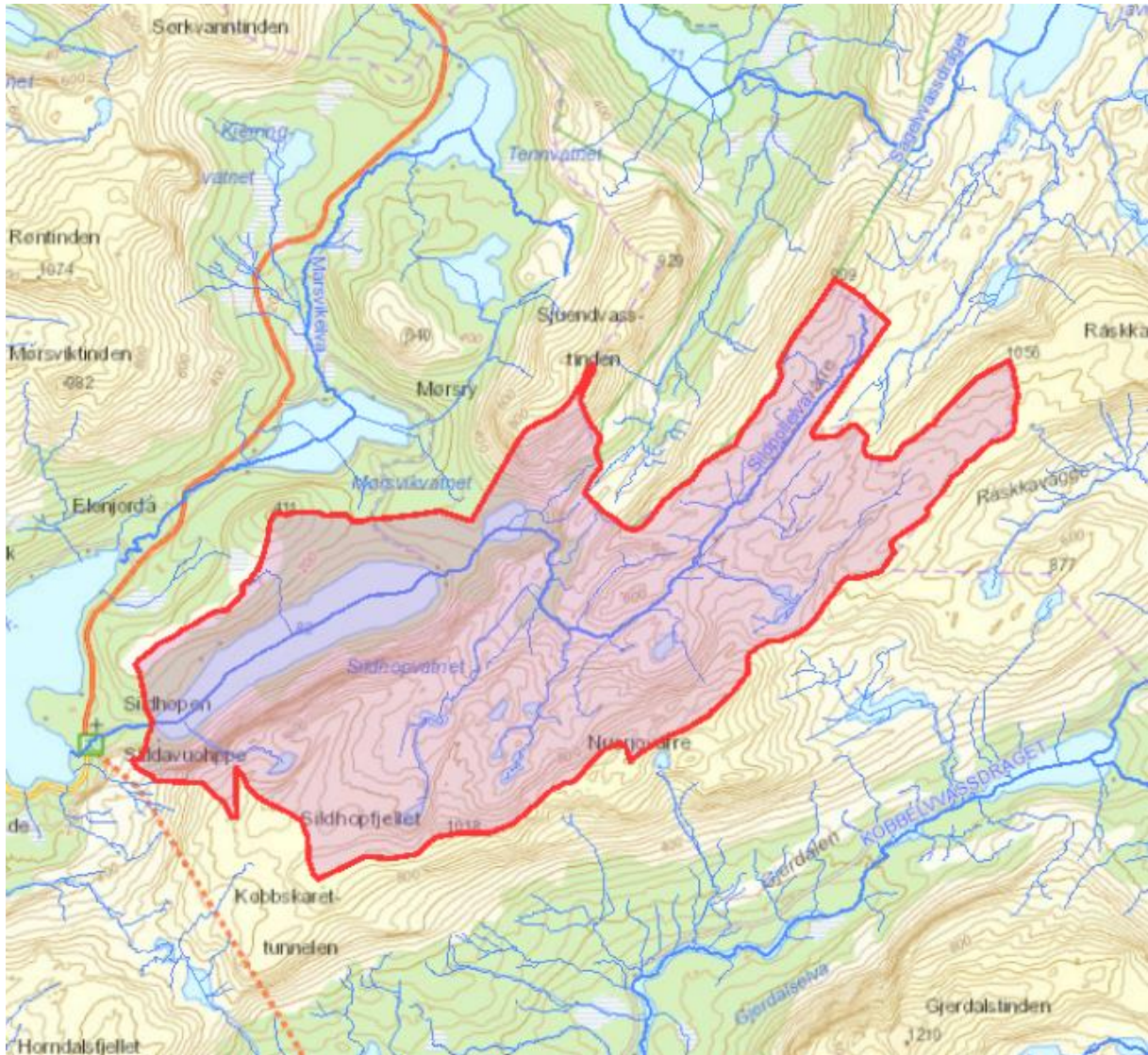
Figur 12 Sildhopen vannverk med nedslagsfelt for Sildhopvatnet
